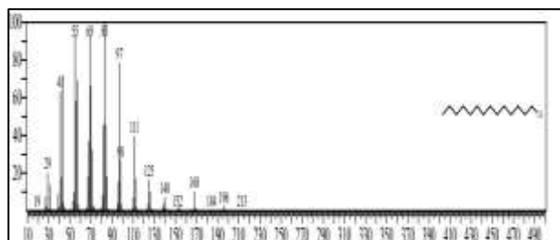
1-Tetradecanol
