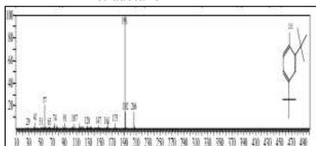
1-Tetradecanol
