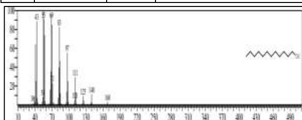
Dodecane
